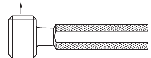
Abnutzungsprüfdorn für Gewindegutleehring Wear testing plug gauge for thread ring gauge Go Mandrin-calibre de vérification d'usure pour bague filetée Entre
